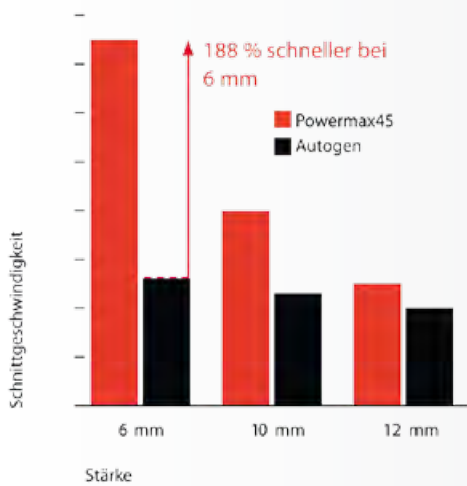
Relative Schneidleistung bei unlegiertem Stahl
